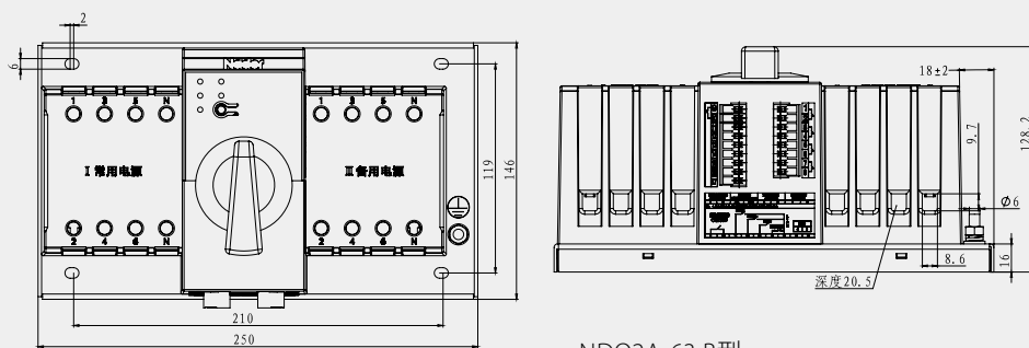
NDQ2A-63 B型
