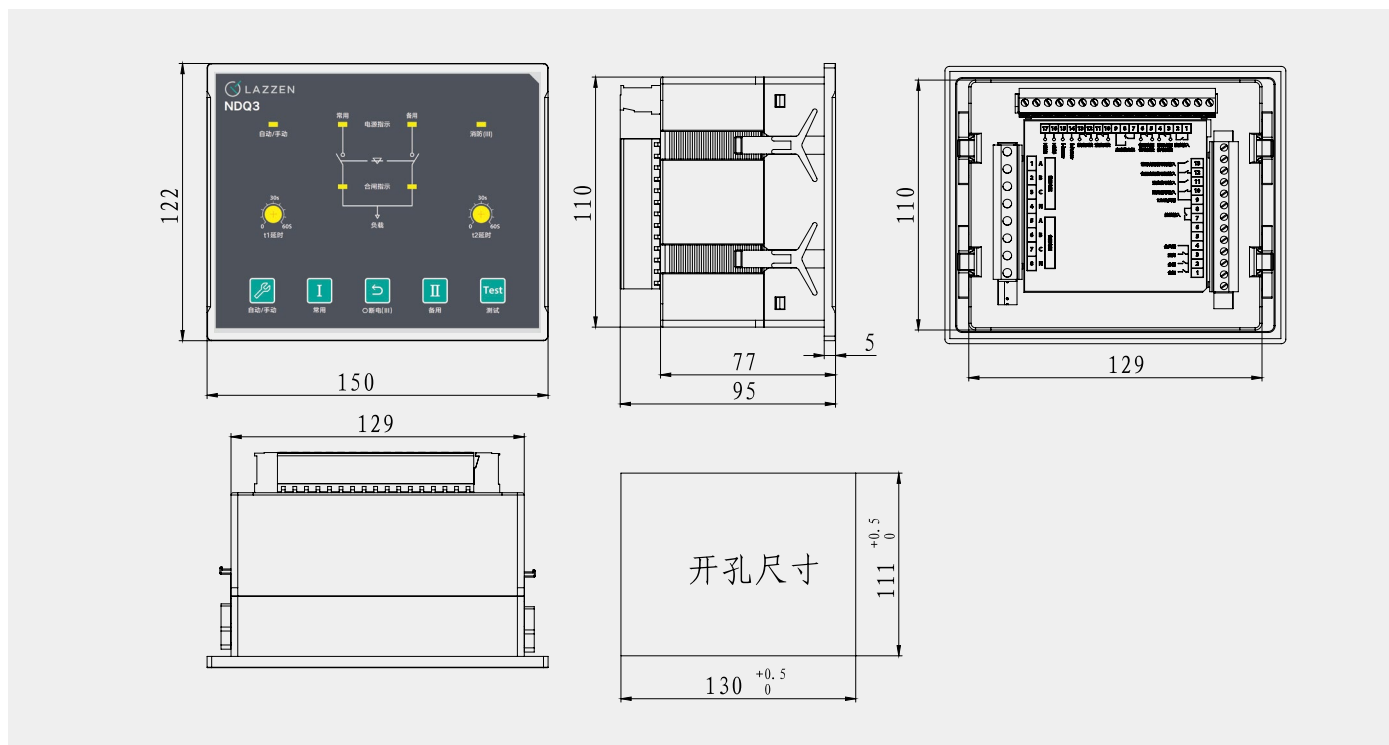
◆ NDQ3-1600壳架N型分体式控制器尺寸图
