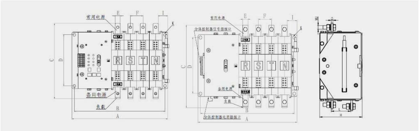
◆ NDQ3两段式250-630整体式/分体式产品尺寸图
