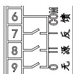
N型分体式 二次端子示意图
