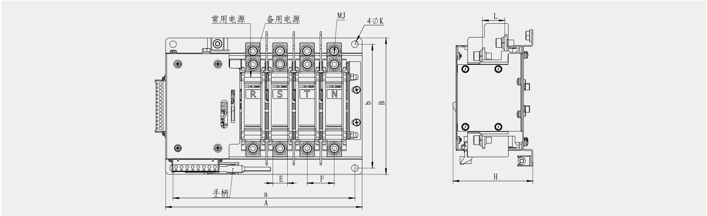
◆ NDQ3两段式125分体产品尺寸图
