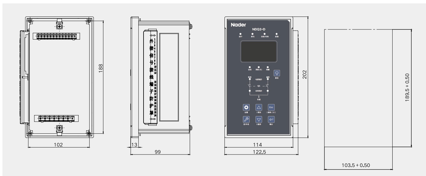
◆ NDQ3-125~800 D型控制器开孔尺寸图
