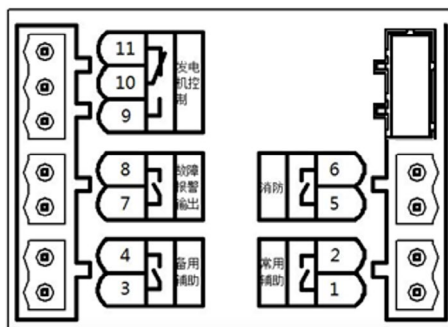
基本型外部端子接线图
