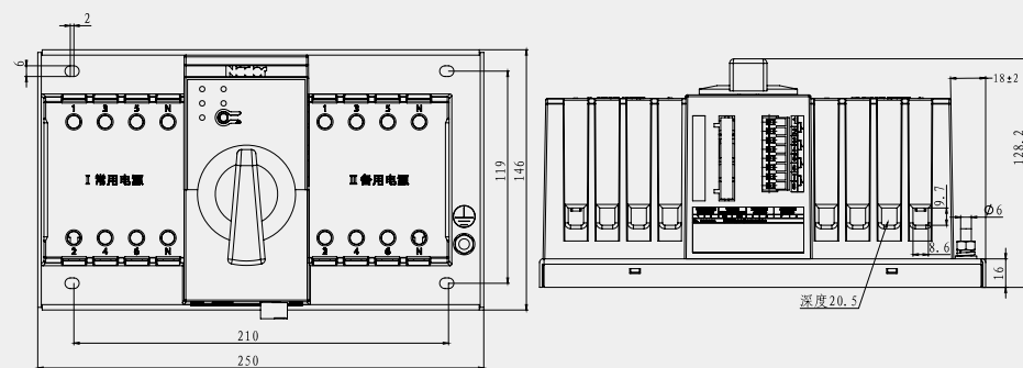
NDQ2A-63 标准型
