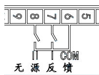
II式空白型分体 二次端子示意图
